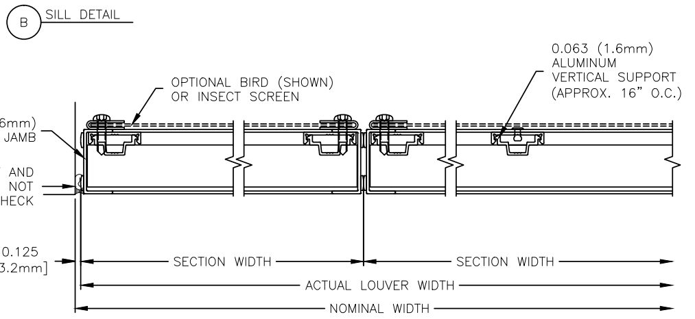
C JAMB DETAIL
