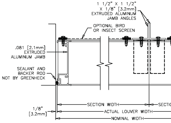
C JAMB DETAIL
