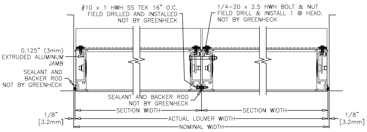
C JAMB DETAIL
