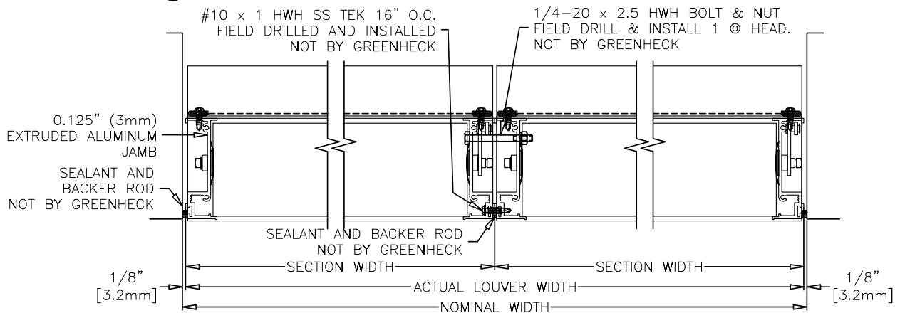
C JAMB DETAIL
